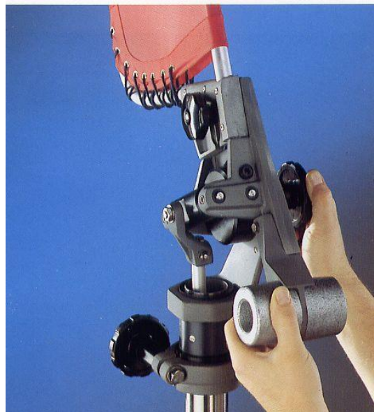
Réglage de l'axe de l'aérien
